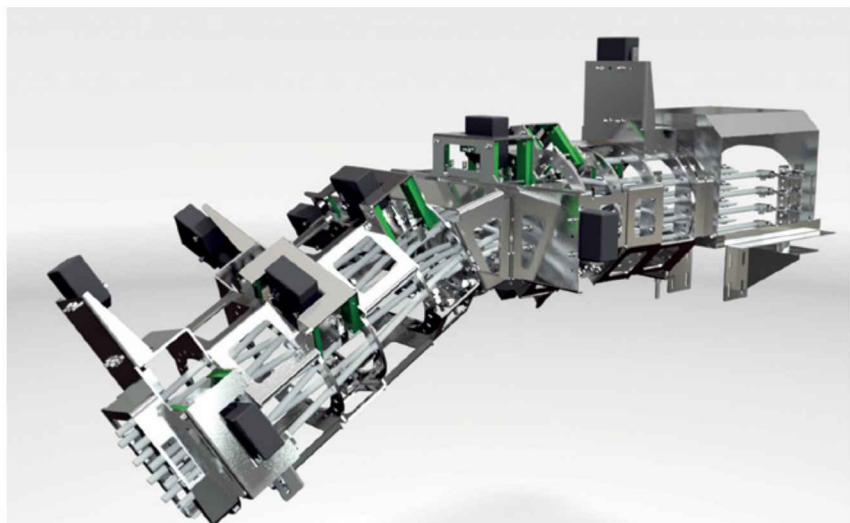
Il sistema Twist automatico vuoti (Magnoni).
